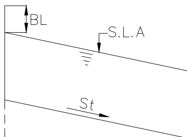
FIGURA 2-6.- Pendiente transversal en una curva
