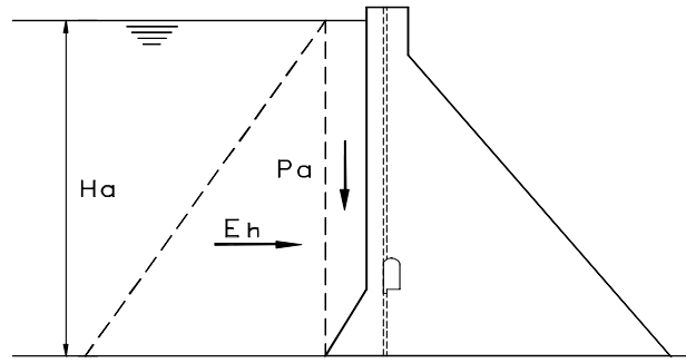
FIGURA 1-4.- Empuje hidrostático.
